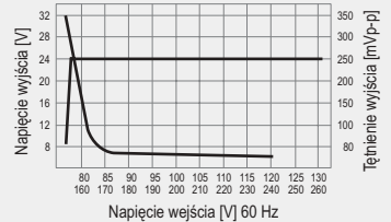
CHARAKTERYSTYKI STATYCZNE (24 V DC) (Ta = 25 °C)
