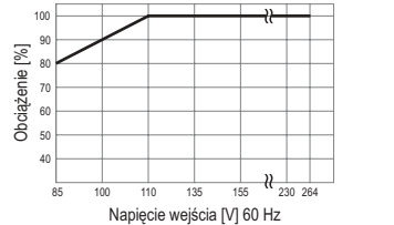
ZALEŻNOŚĆ OBCIĄŻENIA OD NAPIĘCIA WEJŚCIA (Ta = 25 °C)
