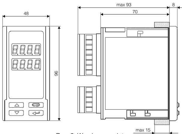
Rys. 2. Wymiary regulatora
