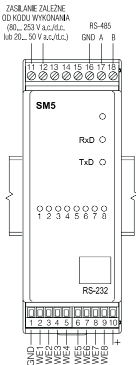
Rys. 2. Podłączenia elektryczne modułu wejść binarnych SM5.
