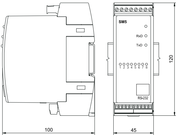
Rys. 1. Rysunek gabarytowy i montażowy.
