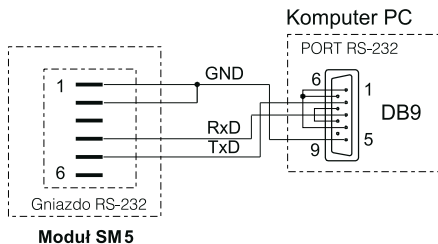
Rys. 4: Sposób podłączenia interfejsu RS-232.
