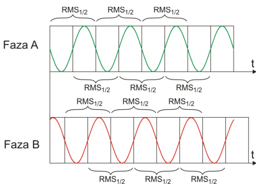
Rys. 20. Wyznaczanie wartości U_{rms(1/2)}
