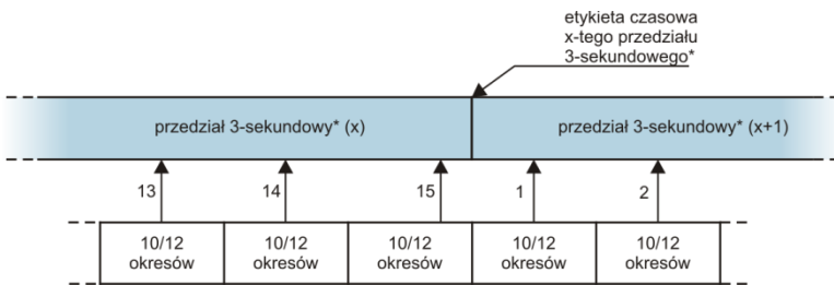
Rys. 23. Wyznaczanie przedziałów uśredniania krótszych od 10 sekund (na przykładzie uśredniania 3-sekundowego)
