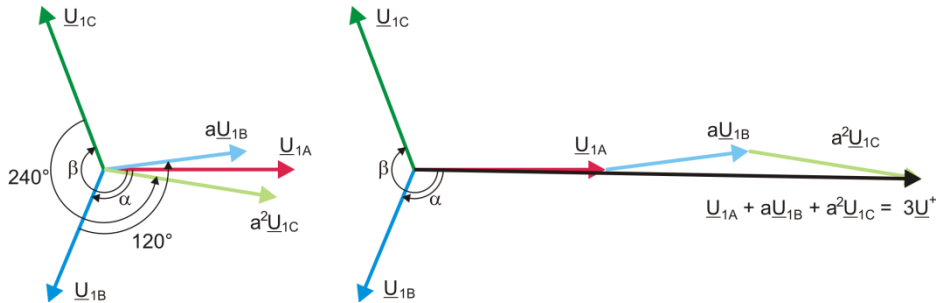
Rys. 18. Przykład wyznaczenia składowej symetrycznej zgodnej.
