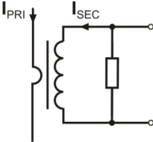
Rys. 16. Cęgi twarde z wyjściem napięciowym
