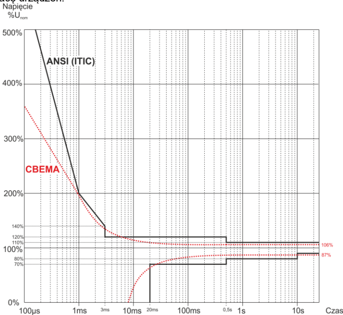
Rys. 21. Krzywe tolerancji napięcia zasilającego ANSI (ITIC) i CBEMA.
