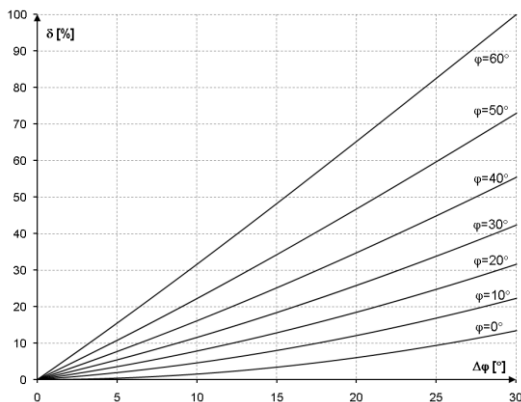
Rys. 24. Niepewność dodatkowa od błęd fazy w zależności od kąta przesunięcia fazowego.
