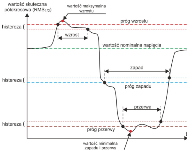
Rys. 19. Wzrosty, zapedy i przerwy napięcia.
