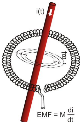
Rys. 17. Cewka Rogowskiego
