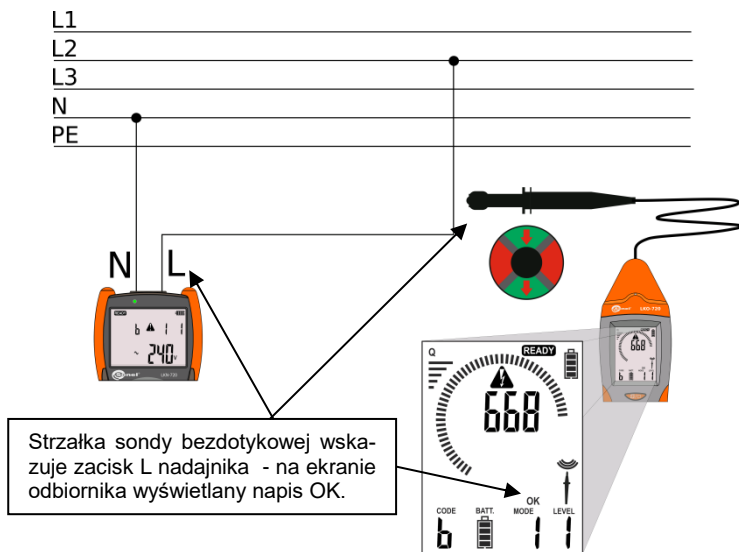
Rys. 41 Sonda bezdotykowa – identyfikacja zacisku L nadajnika.
