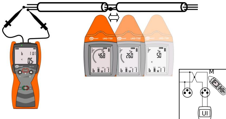
Rys. 26 Lokalizacja zwarcia żył w przewodzie.
