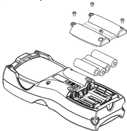
Rys. 16 Nadajnik – wymiana baterii.
