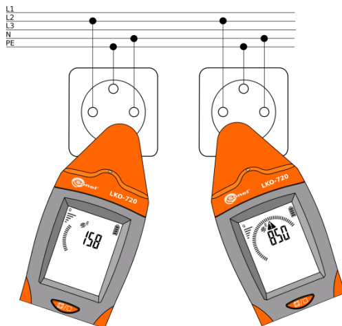
Rys. 32 Wykrywanie pola elektrycznego.
