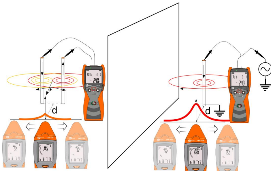
Rys. 18 Wektory pola magnetycznego w dwóch równoległych przewodach.
