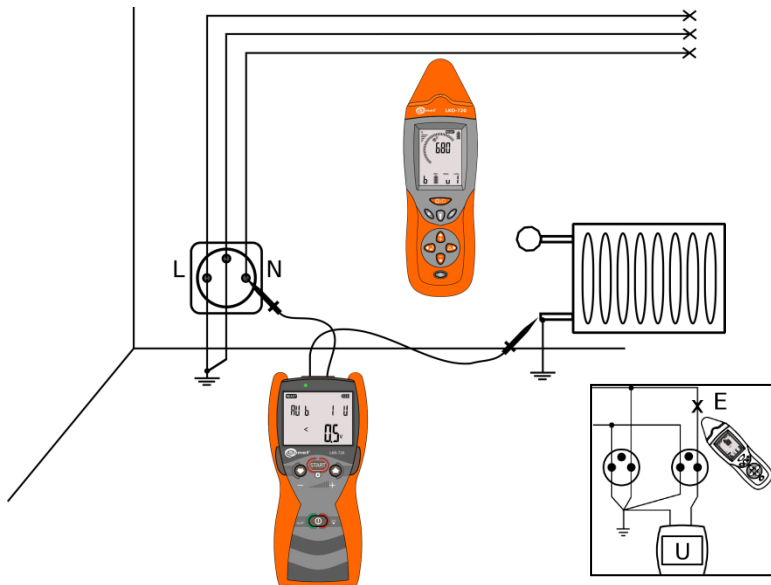
Rys. 23 Lokalizacja przewodów w ścianie odłączonych od sieci.
