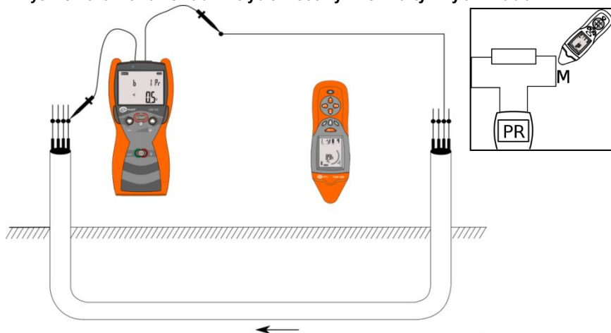
Rys. 29 Lokalizowanie kabli w trybie mocowym z użyciem przewodu zewnętrznego.
