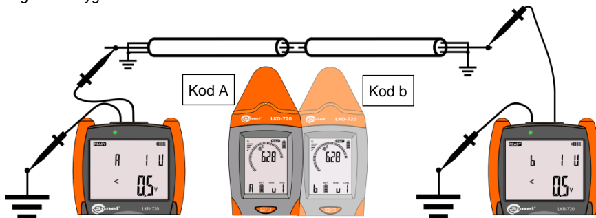
Rys. 33 Lokalizacja przerw – tryb wielonadajnikowy.
