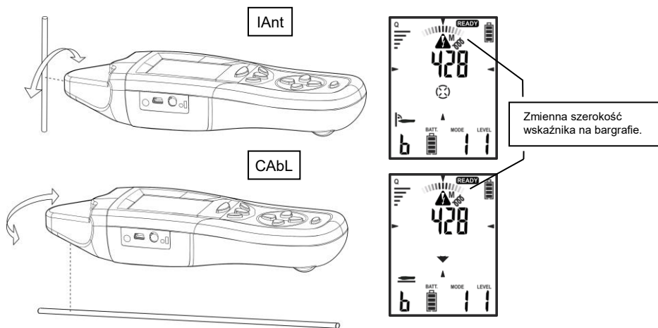
Rys. 22 Szerokość wskaźnika na bargrafie
