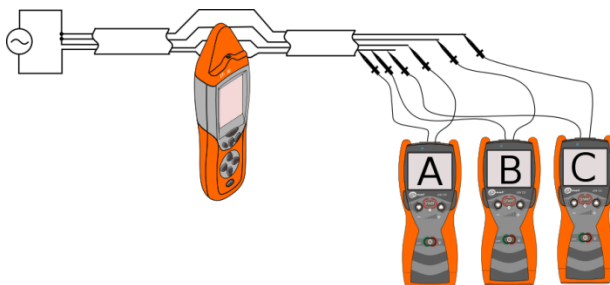
Rys. 34 Identyfikacja żył w przewodzie – tryb I.
