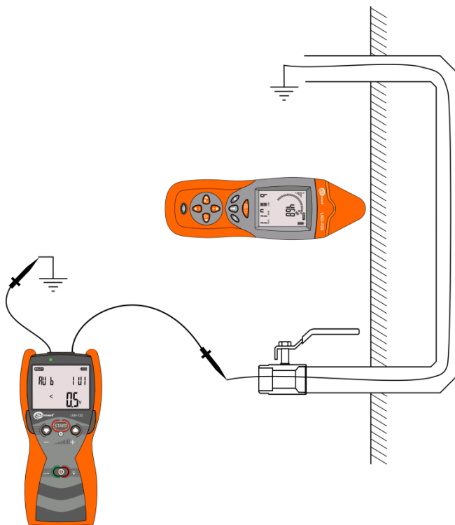
Rys. 30 Lokalizacja nieprzewodzącej elektrycznie instalacji hydraulicznej.
