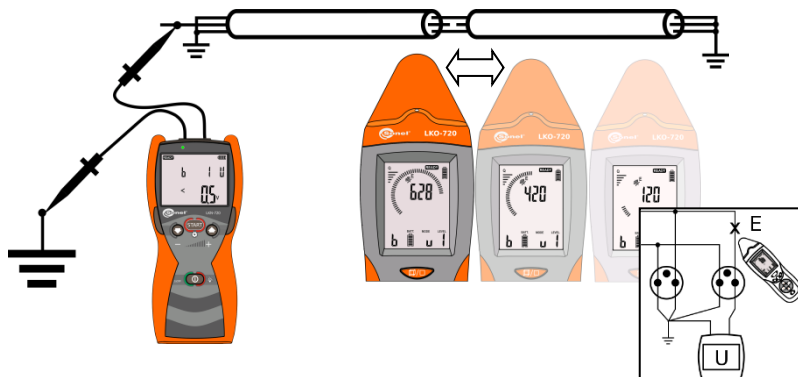
Rys. 25 Lokalizacja przerwy.
