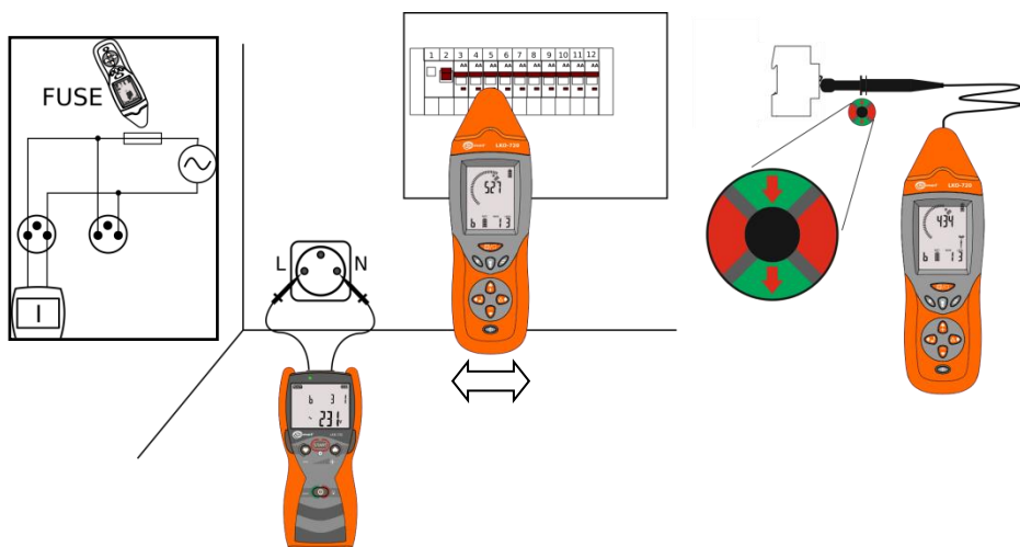
Rys. 27 Identyfikacja zabezpieczeń w rozdzielnicy.
