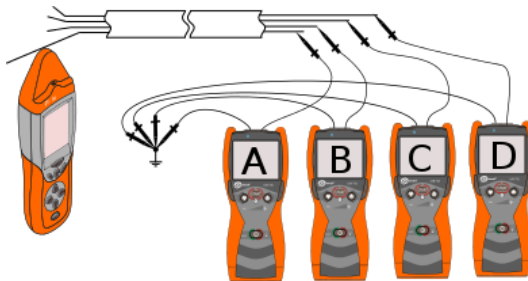
Rys. 35 Identyfikacja żył w przewodzie – tryb U.
