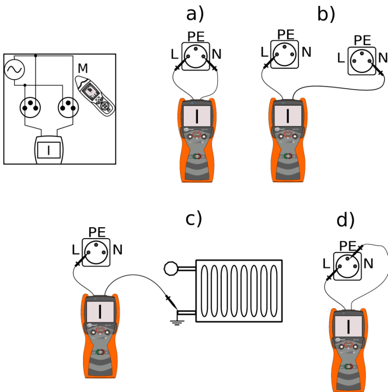
Rys. 17 Przykłady podłączenia nadajnika do instalacji elektrycznej.
