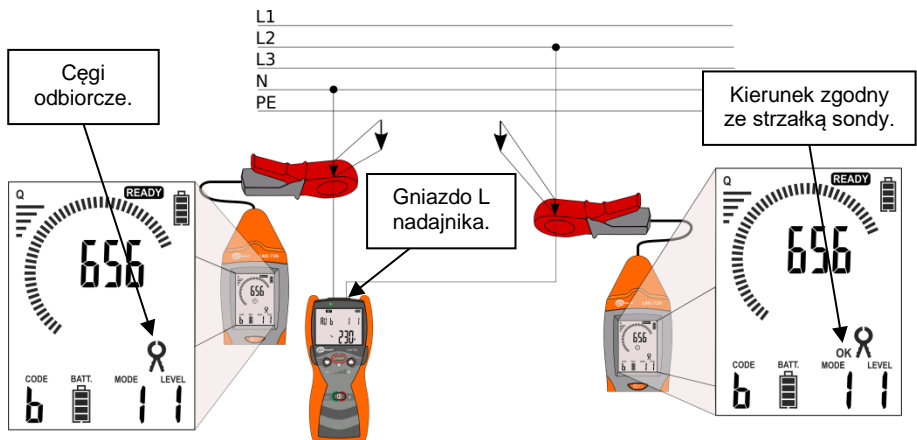
Rys. 37 Cęgi odbiorcze – wymuszenie prądowe w lokalizowanym obwodzie.
