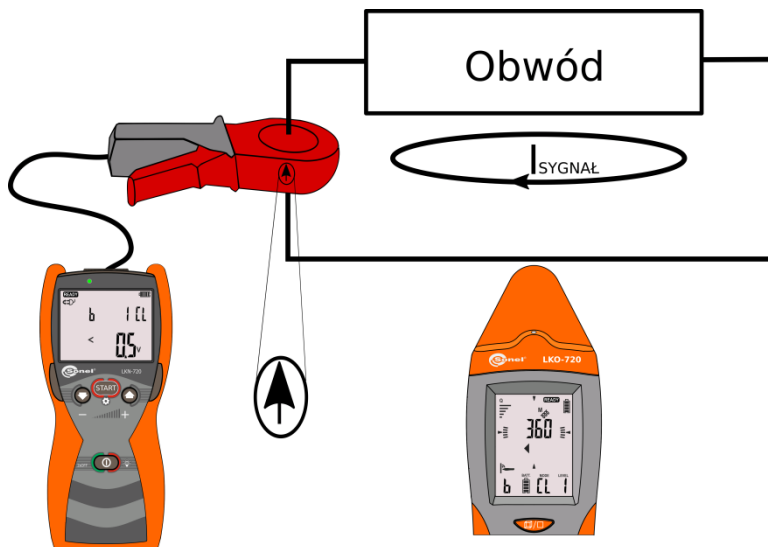
Rys. 36 Cęgi nadawcze – wymuszenie prądowe w lokalizowanym obwodzie.
