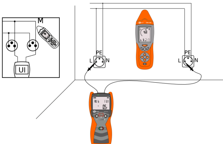
Rys. 24 Lokalizacja instalacji elektrycznej wykorzystująca zamkniętą pętlę.
