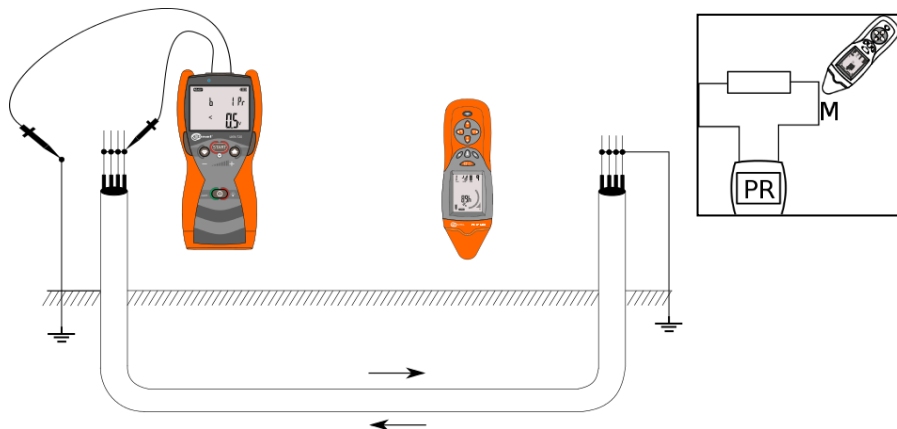
Rys. 28 Lokalizowanie kabli w trybie mocowym ze zwartym żyłami kabla.
