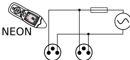
Rys. 14 Schemat trybu wykrywania pola elektrycznego 50Hz/60Hz.
