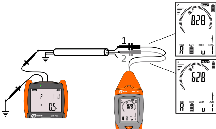
Rys. 38 Sonda dotykowa – identyfikacja przewodów.
