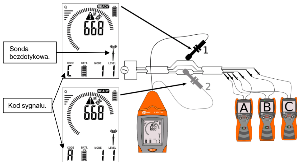
Rys. 40 Sonda bezdotykowa – identyfikacja przewodów przy pracy wielonadajnikowej.
