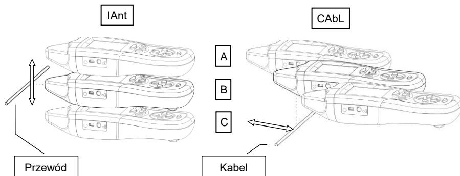
Rys. 19 Lokalizacja przewodu / kabla położonego prostopadłe do osi symetrii odbiornika.
