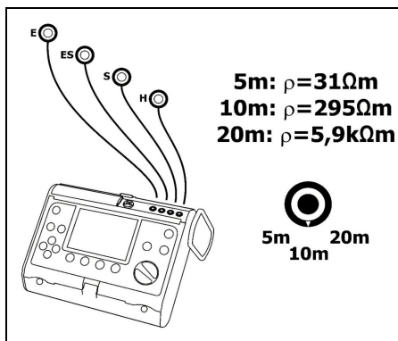
Rys.15. Podłączenie miernika.
