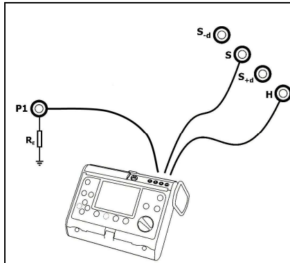
Rys.7. Podłączenie miernika.
