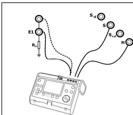
Rys.8. Podłączenie miernika.
